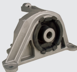
Suporte do Câmbio Lado Esquerdo
